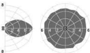
Активная зона действия датчика
