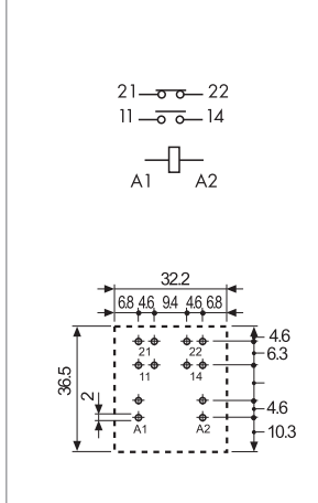
Вид со стороны выводов
