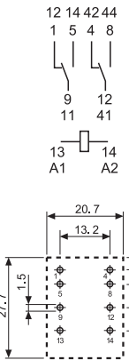
Вид со стороны выводов
