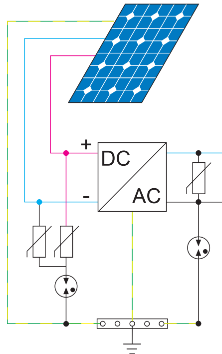
Рис 10: пример фотovoltaической системы для здания не оборудованного системой защиты от молнии; защита со стороны DC при помощи УЗИП с U_{oc stc} = 420 В, и защита со стороны AC устройством 7P.22, характерным для систем TT.
