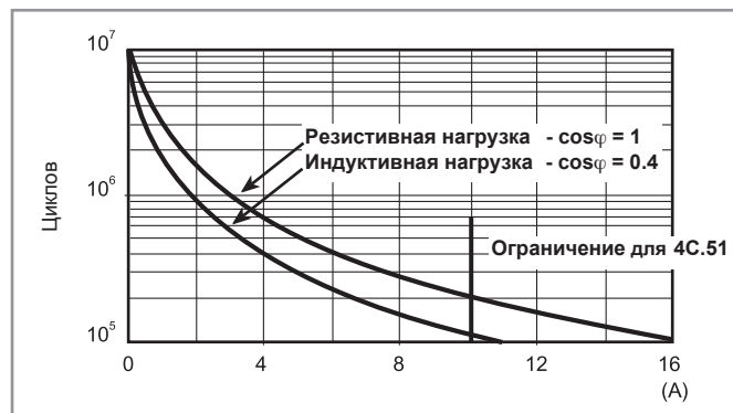
F 4C - Электрическая долговечность (AC) при ном. нагрузке, Типы 4C.01/51
