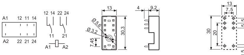
Вид со стороны выводов
