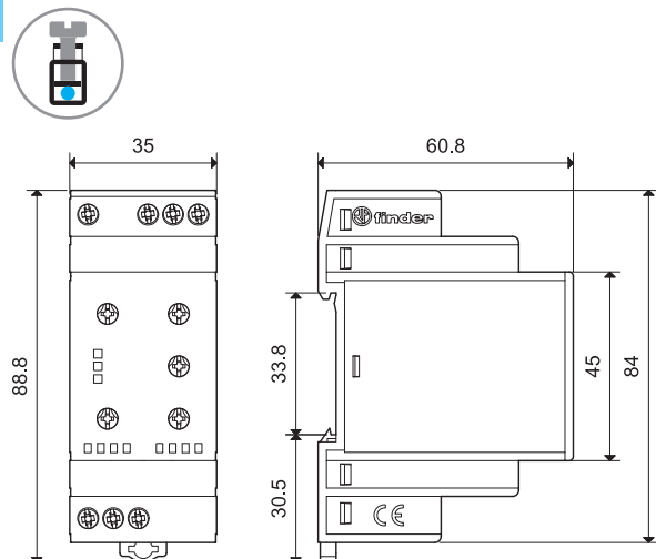
E 70.41 Винтовой зажим
