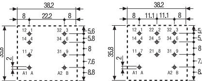
62.22 62.23 Вид со стороны выводов
