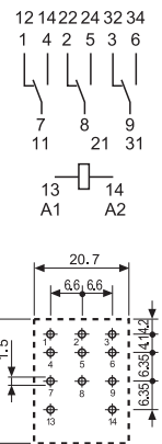
Вид со стороны выводов
