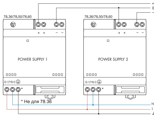
последовательное соединение
