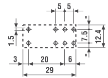
Вид со стороны выводов
