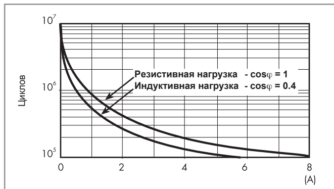
F 49 - Электрическая долговечность (AC) при ном. нагрузке, Типы 49.52/72
