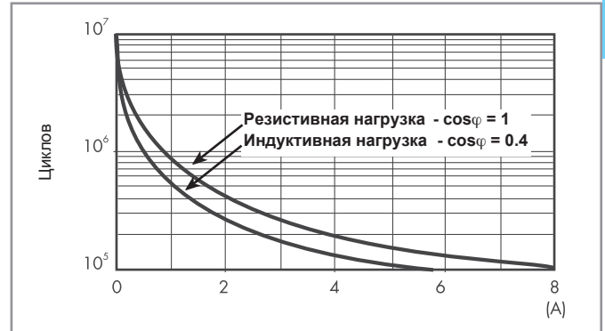
F 40 - Электрическая долговечность (AC) при ном. нагрузке Типы 40.52
