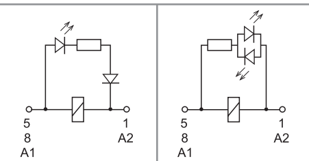
C: Опция 54 светодиод (AC) C: Опция 74 СИД (неполяризованный DC)
