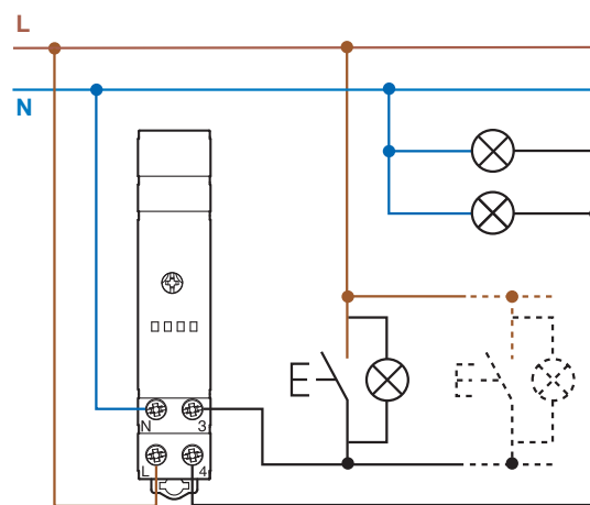
4-проводное соединение
