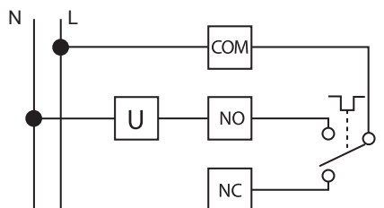
Электрическая принципиальная схема
