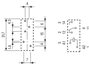
Вид со стороны выводов
