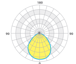
КСС ТИП «Д»
