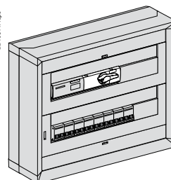
Выключатель-разъединитель Compact INS40 на DIN-рейке
