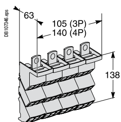
Распределительный блок Linergy DP 250 А
