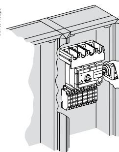
Установка в кабельном канале шириной 300 мм
