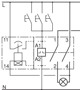
Таймер ATLt + импульсное реле TL
