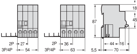
Vigi C60 25A
