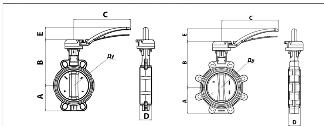
VFY с металлической рукояткой
